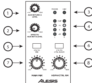
SECTION PRINCIPALE
